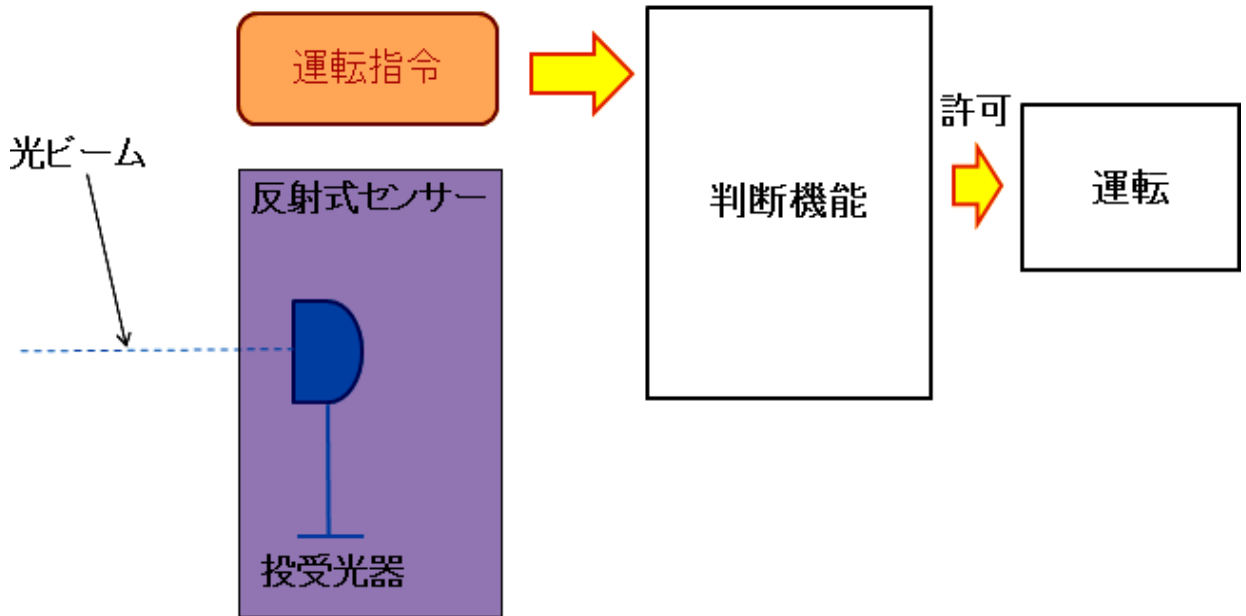
図4-13 危険検出型システム(2)
